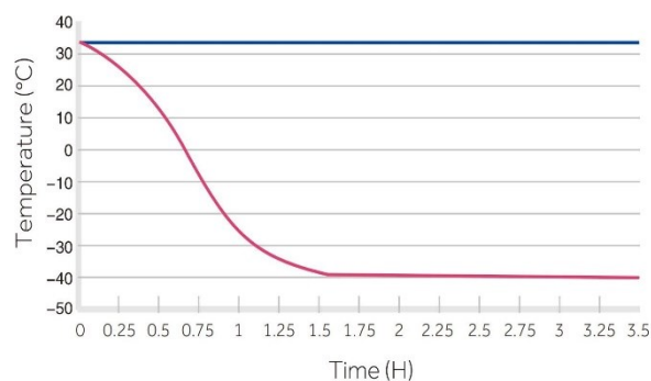
Curva descenso de temperatura ambiente
